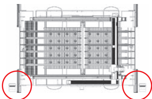
Master 53-55 e 63-65 di serie comprendono doppi comandi macchina posti alle due estremità del centro di lavoro per offrire la massima comodità all'operatore. Nella foto configurazione speciale con armadio anteriore a destra. Nel lay out configurazione standard.
