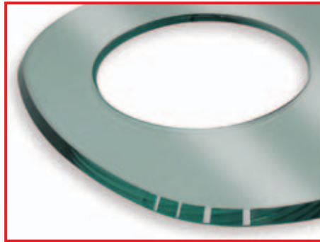
Esempio di profilo smussato a 45° con molatura a tazza.
